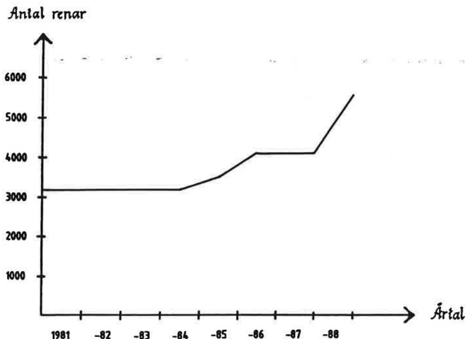
Diagram 2. Antal renar inom Tåssåsens sameby under åren 1981-1988
