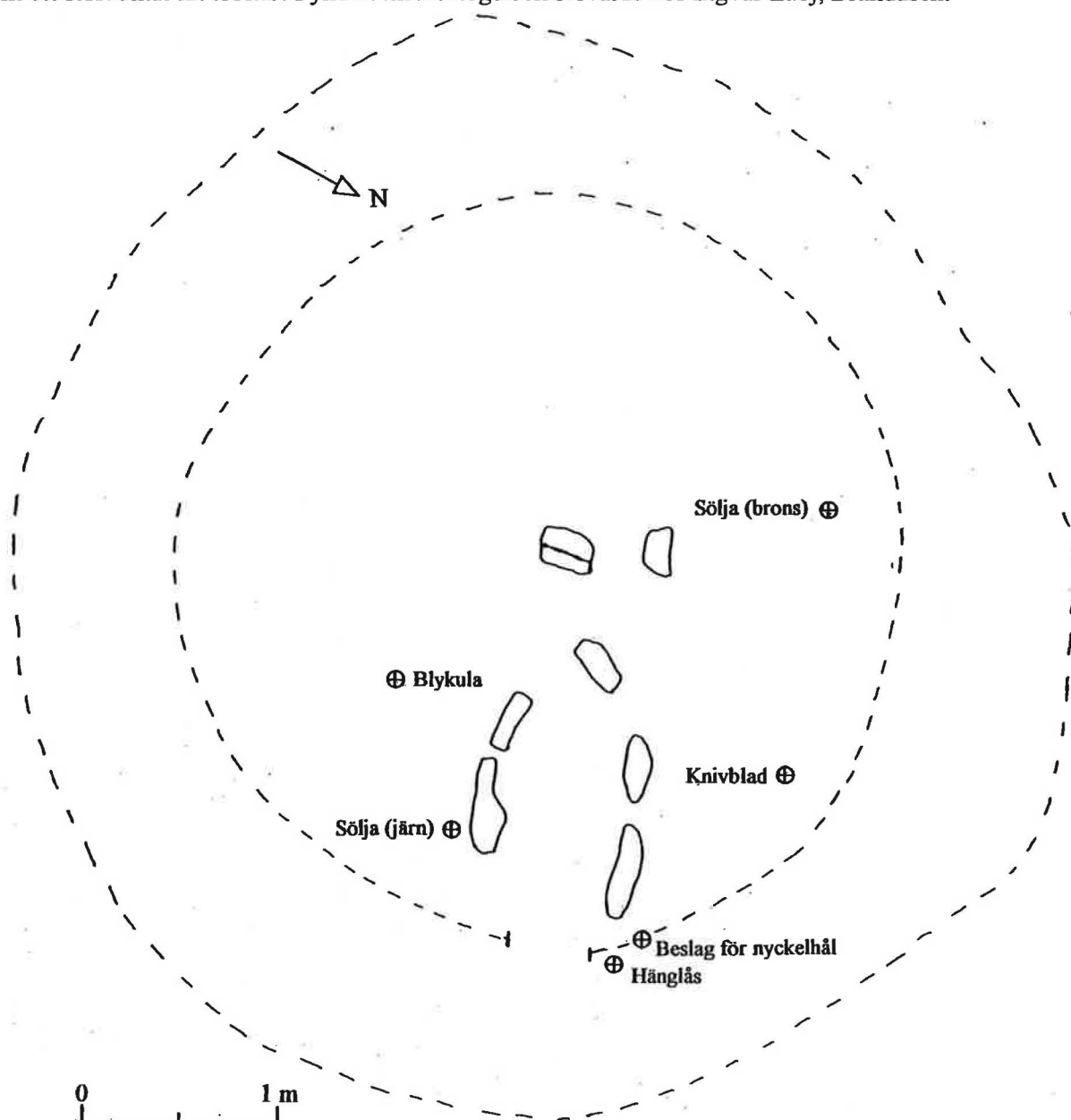
Fig. 3. Myskelsjön. Kåtatomten markeras med en 1 – 1,5 m bred vall. Två parallella stenarmar går mot ingången som även markeras av en svacka i vallen. Ritning Sven-Donald Hedman.
