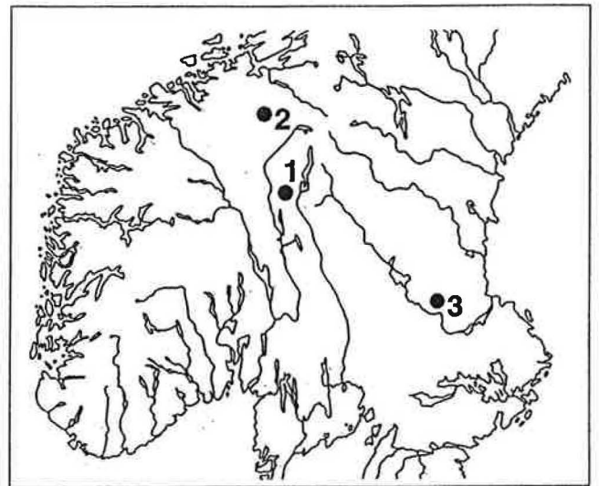
Fig. 110. Platser med fynd vittnande om rituella bruk nämnda i texten. Vikingatid-medeltid. 1. Øvre Rendalen. 2. Finntjønnan. 3. Sundbornsmossen.
